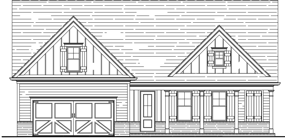
ELEVATION A
